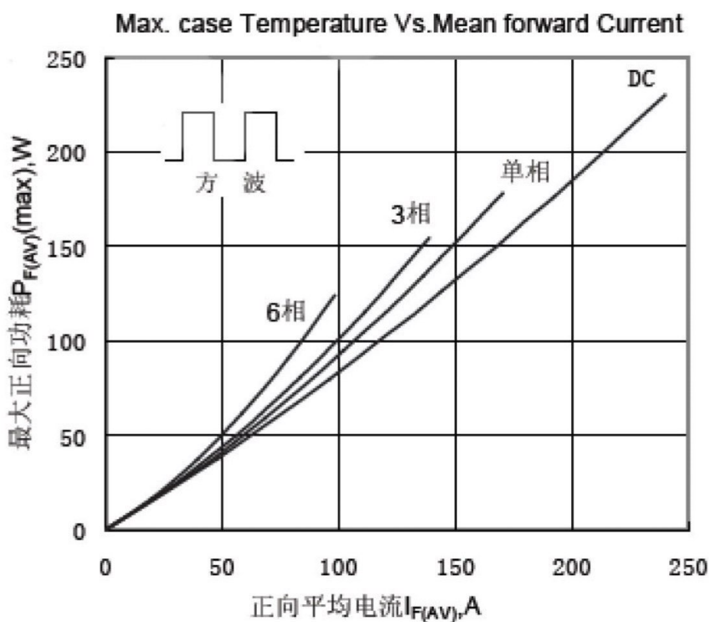
Fig.5 最大正向功耗与平均电流关系曲线
