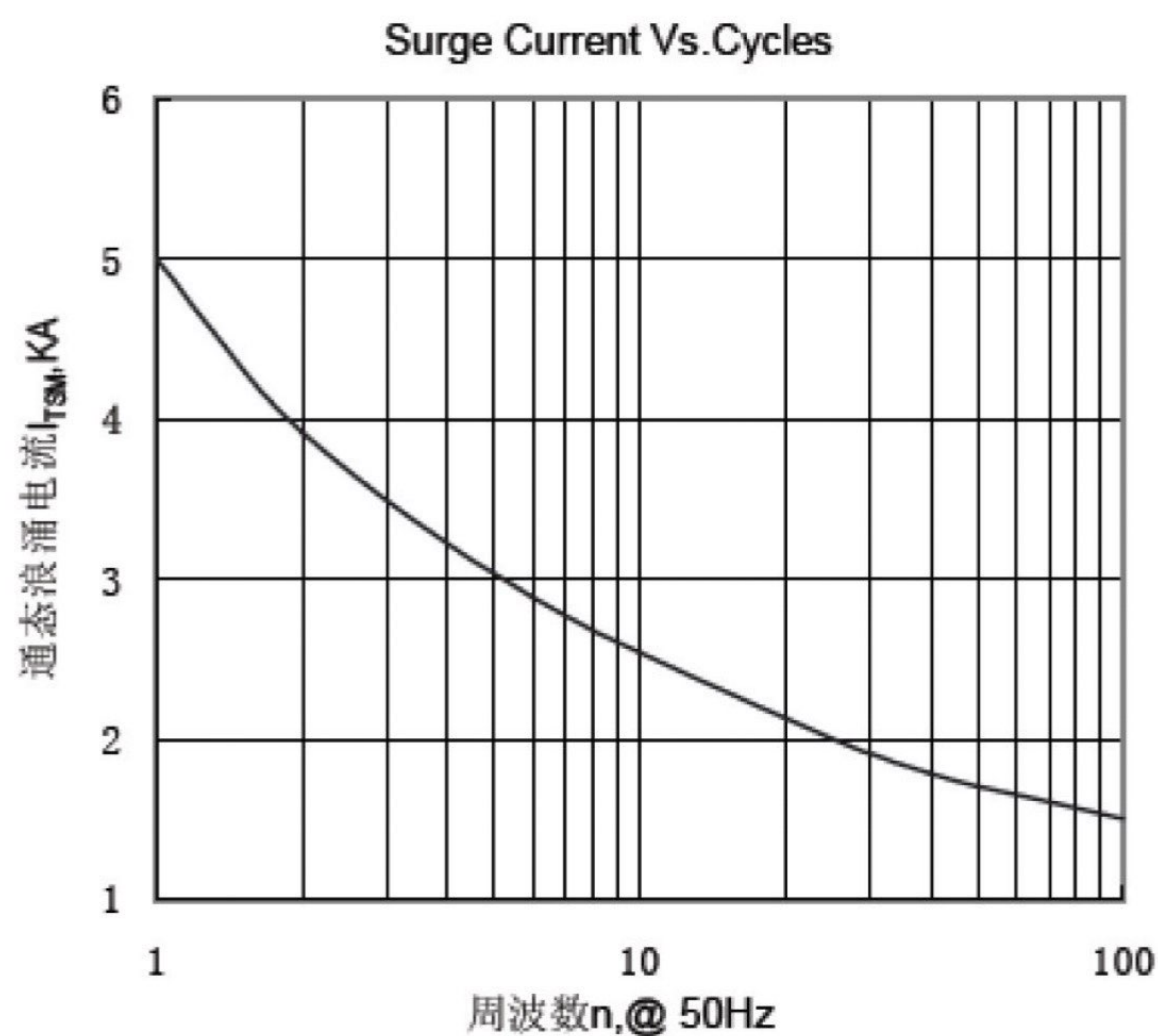
Fig.7 通态浪涌电流与周波数的关系曲线
