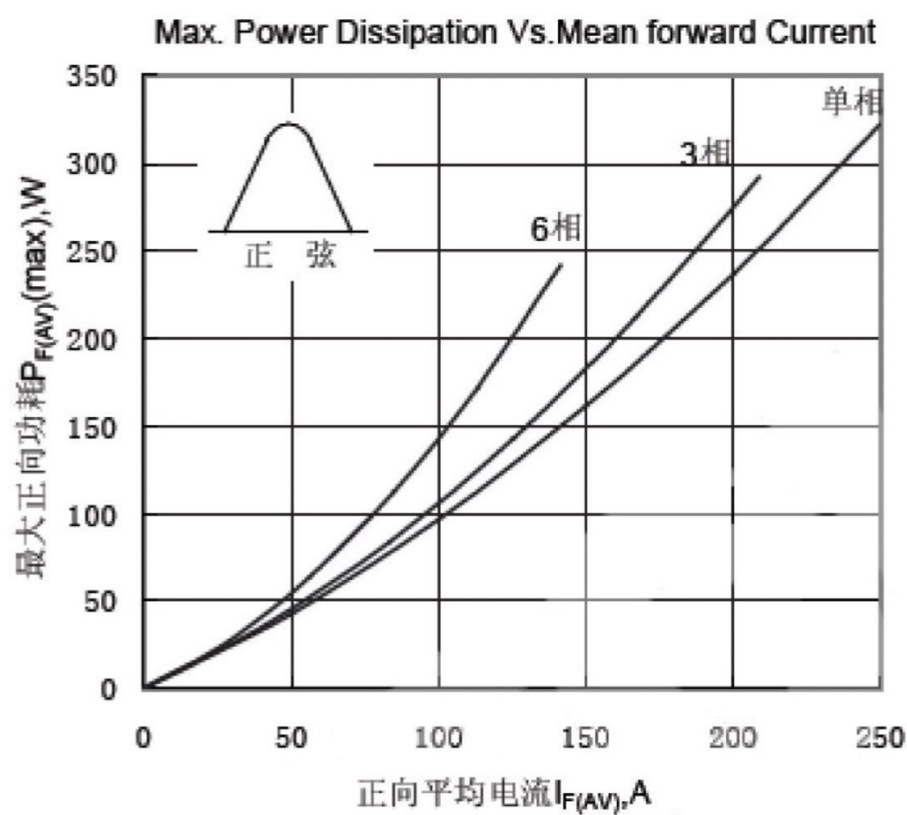
Fig.3 最大正向功耗与平均电流关系曲线
