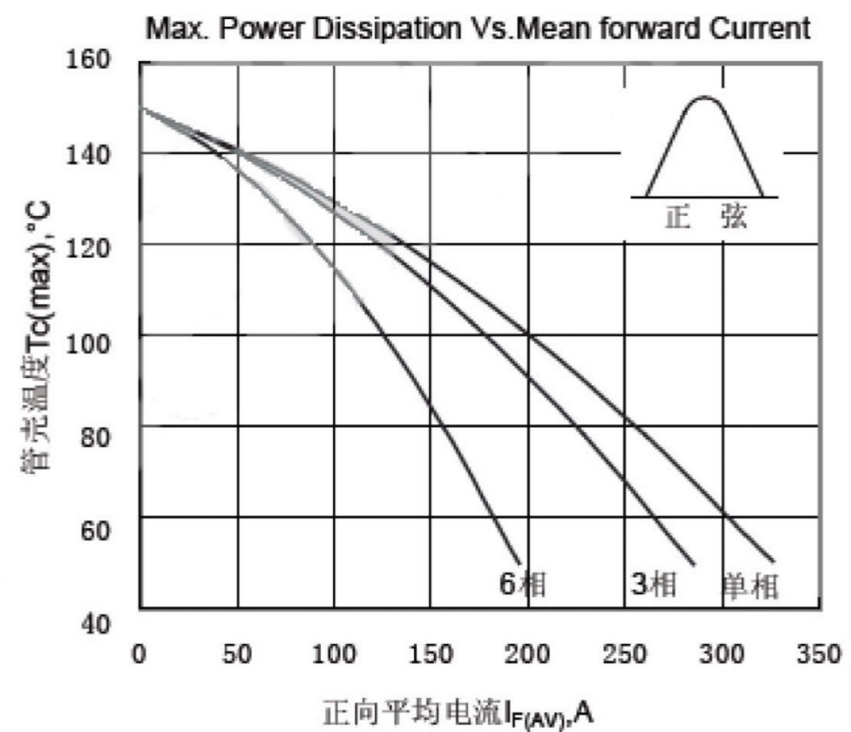
Fig.4 管壳温度与正向平均电流关系曲线
