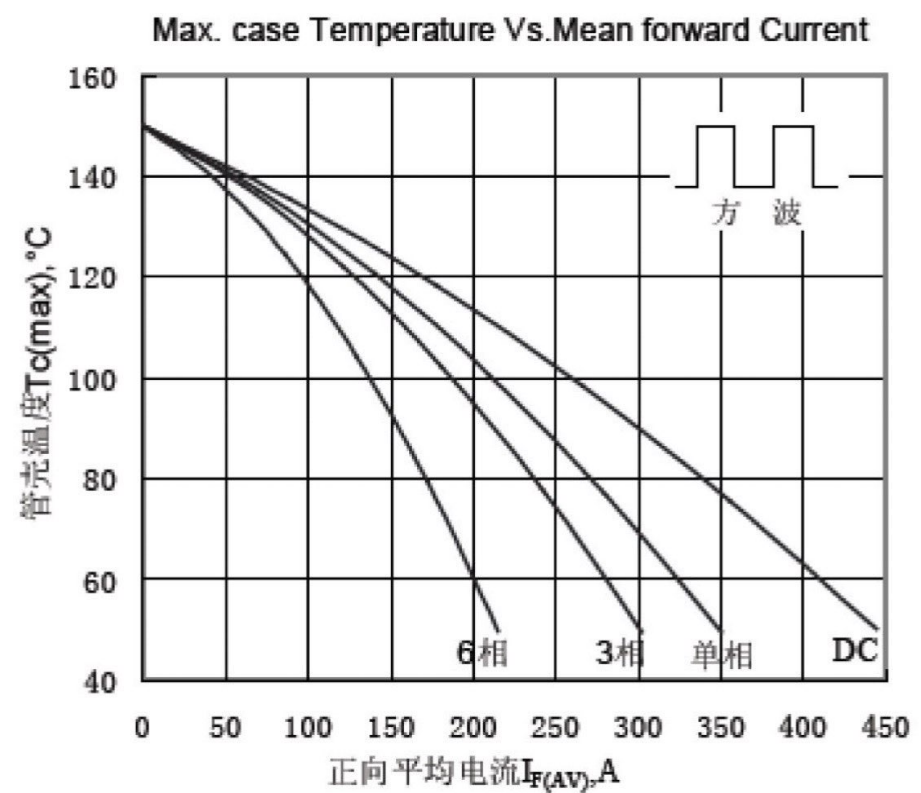
Fig.6 管壳温度与正向平均电流关系曲线
