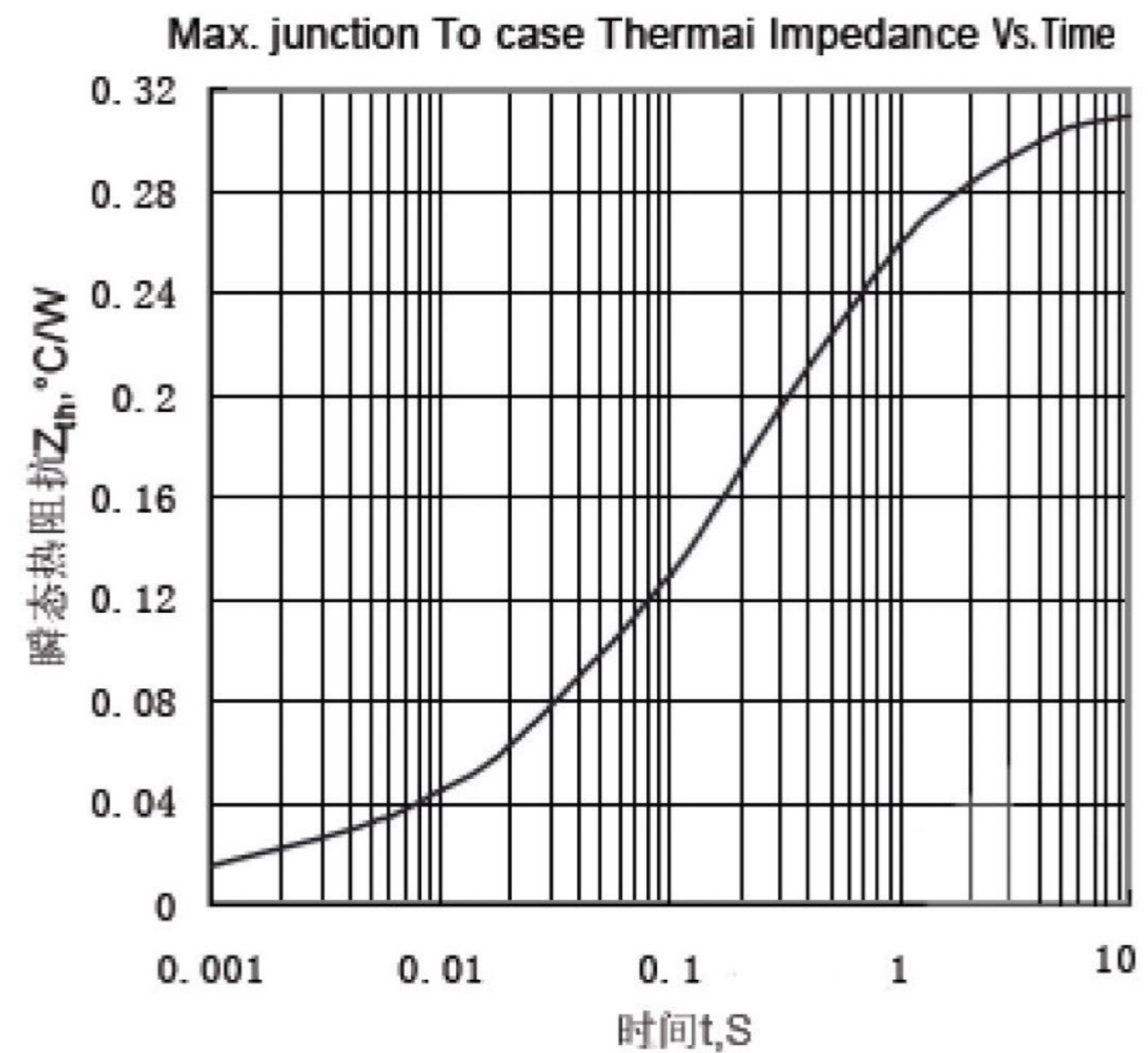
Fig.2 瞬态热阻抗曲线
