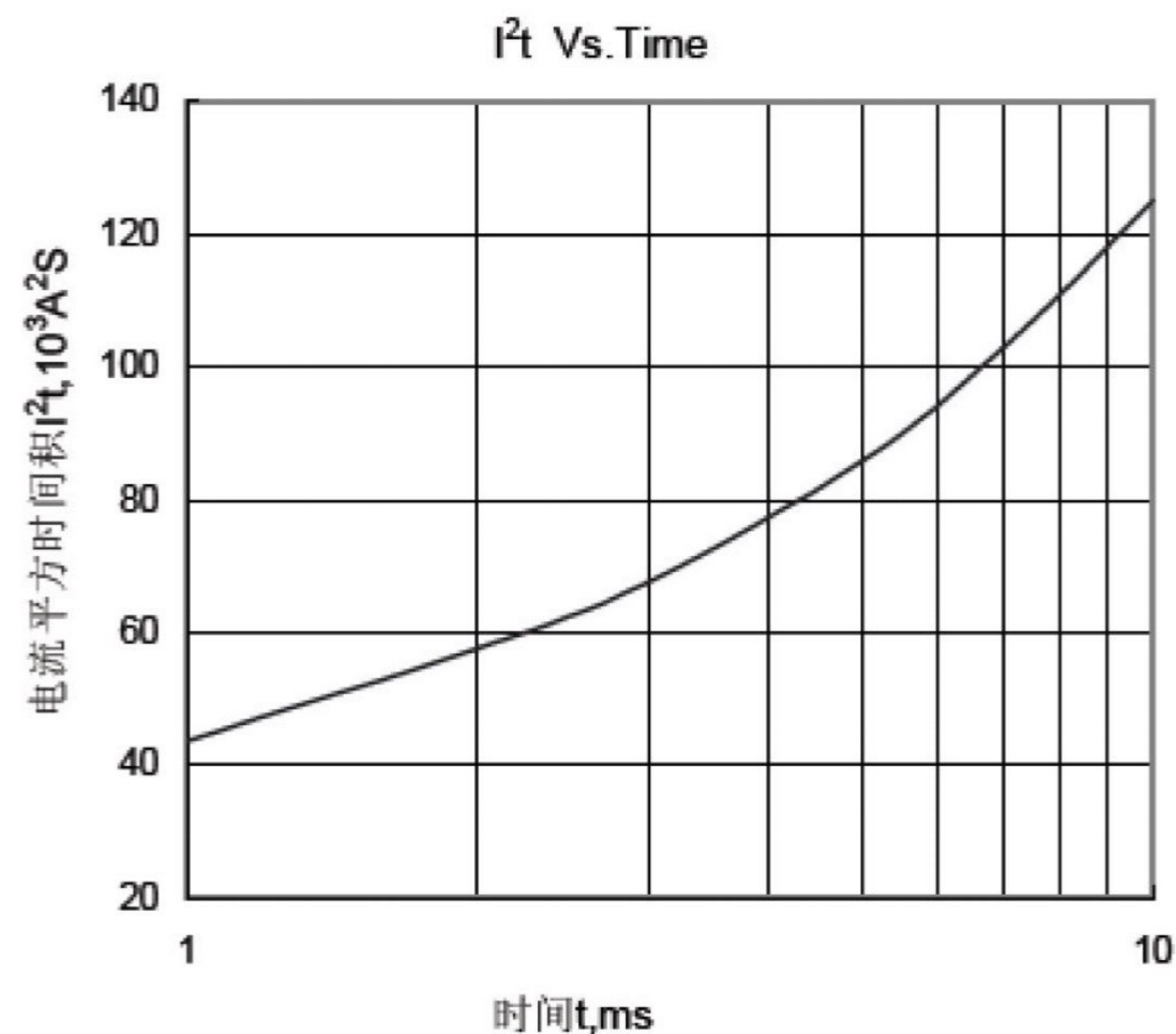
Fig.8 I^2t 特性曲线
