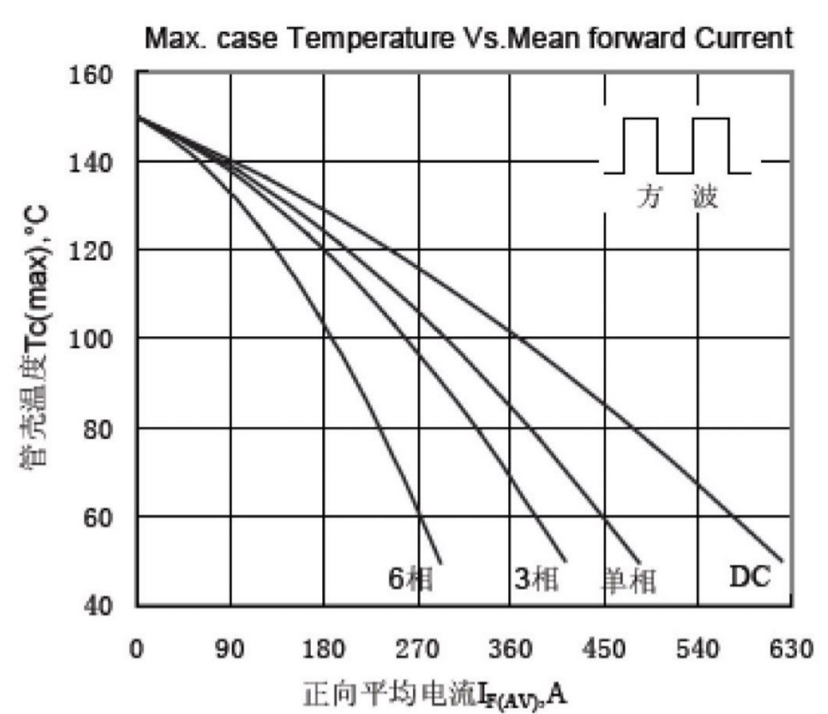
Fig.6 管壳温度与正向平均电流关系曲线
