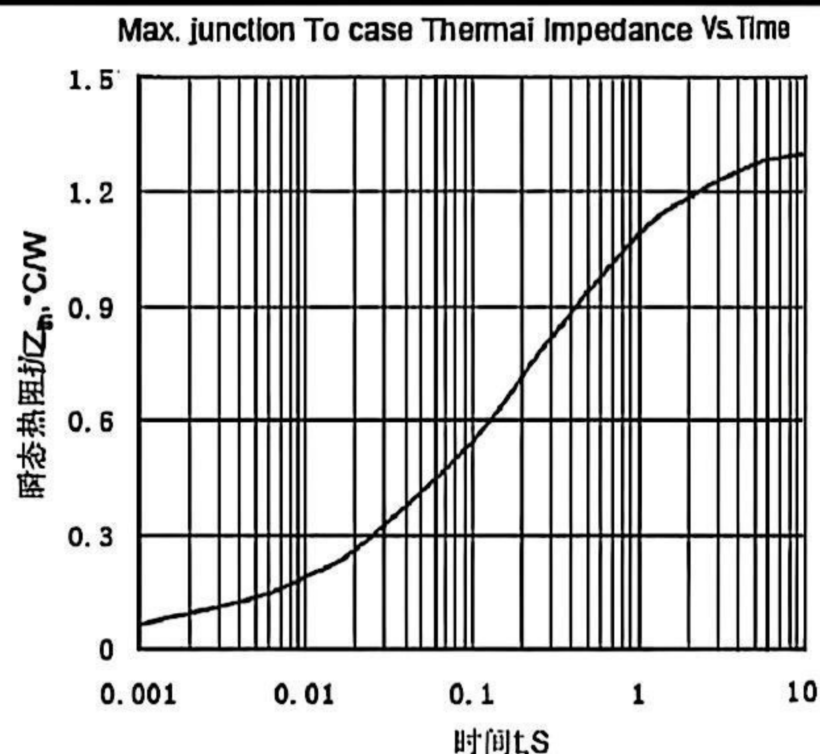
Fig.2 瞬态热阻抗曲线
