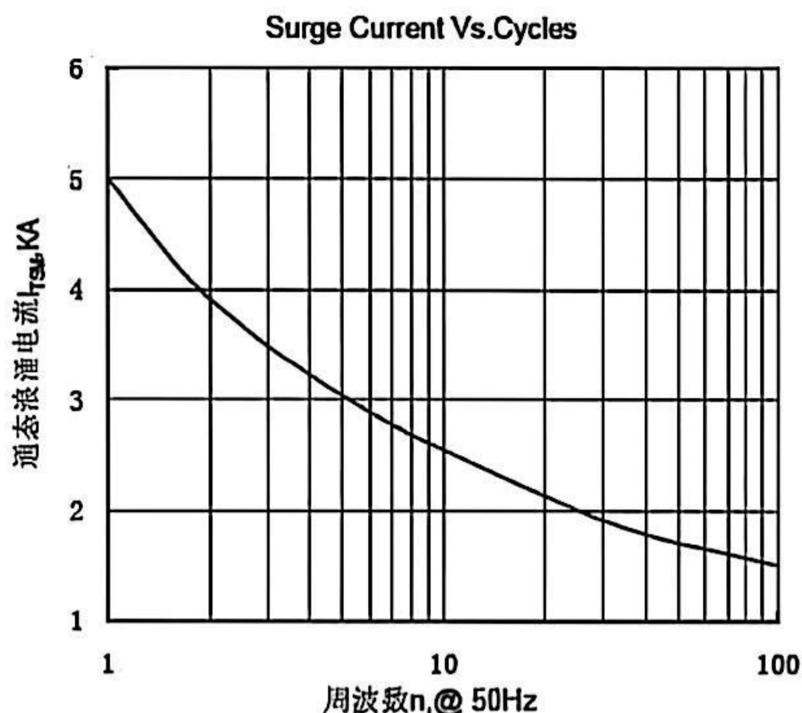
Fig.7 通态浪涌电流与周波数的关系曲线
