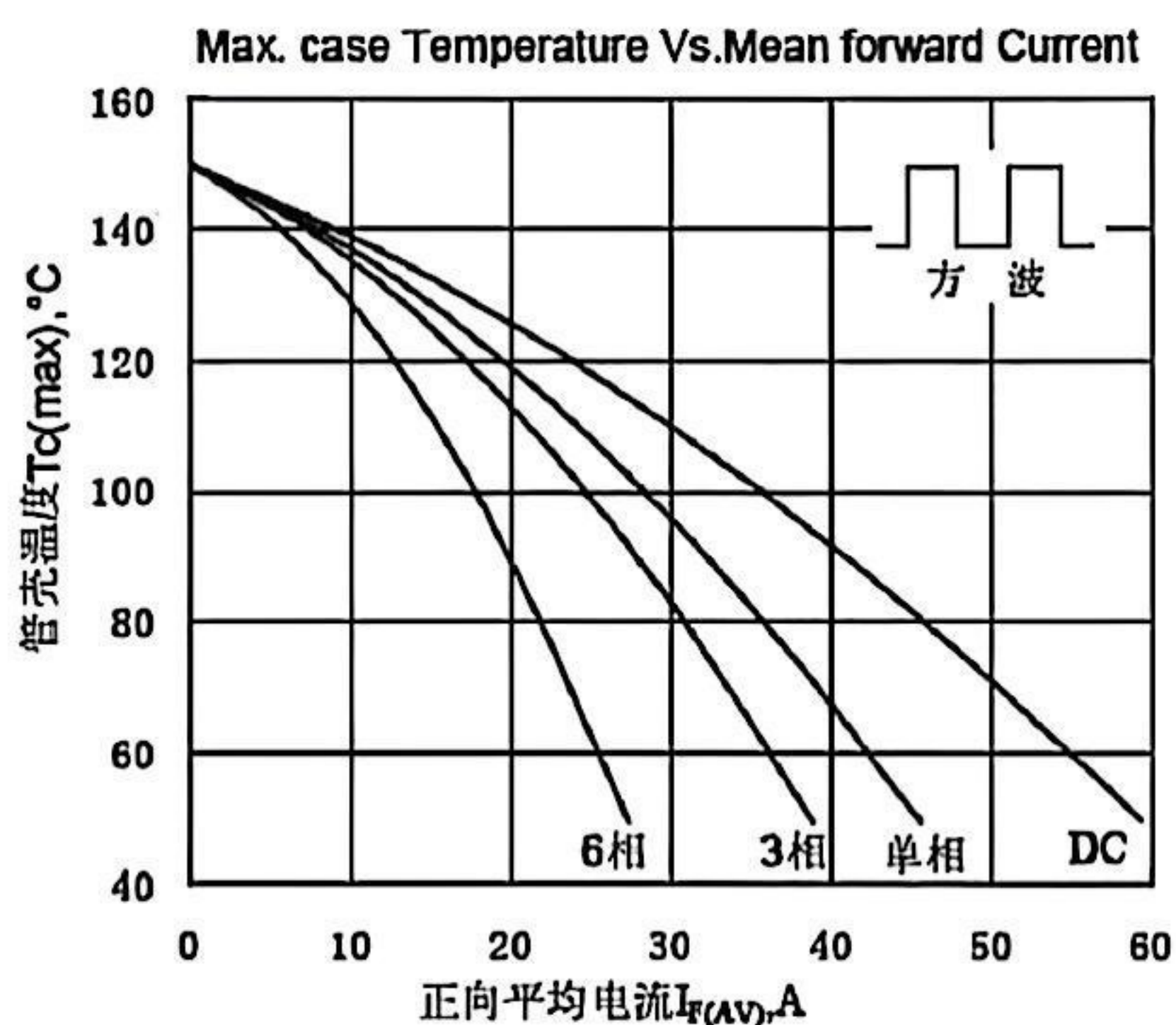
Fig.6 管壳温度与正向平均电流关系曲线
