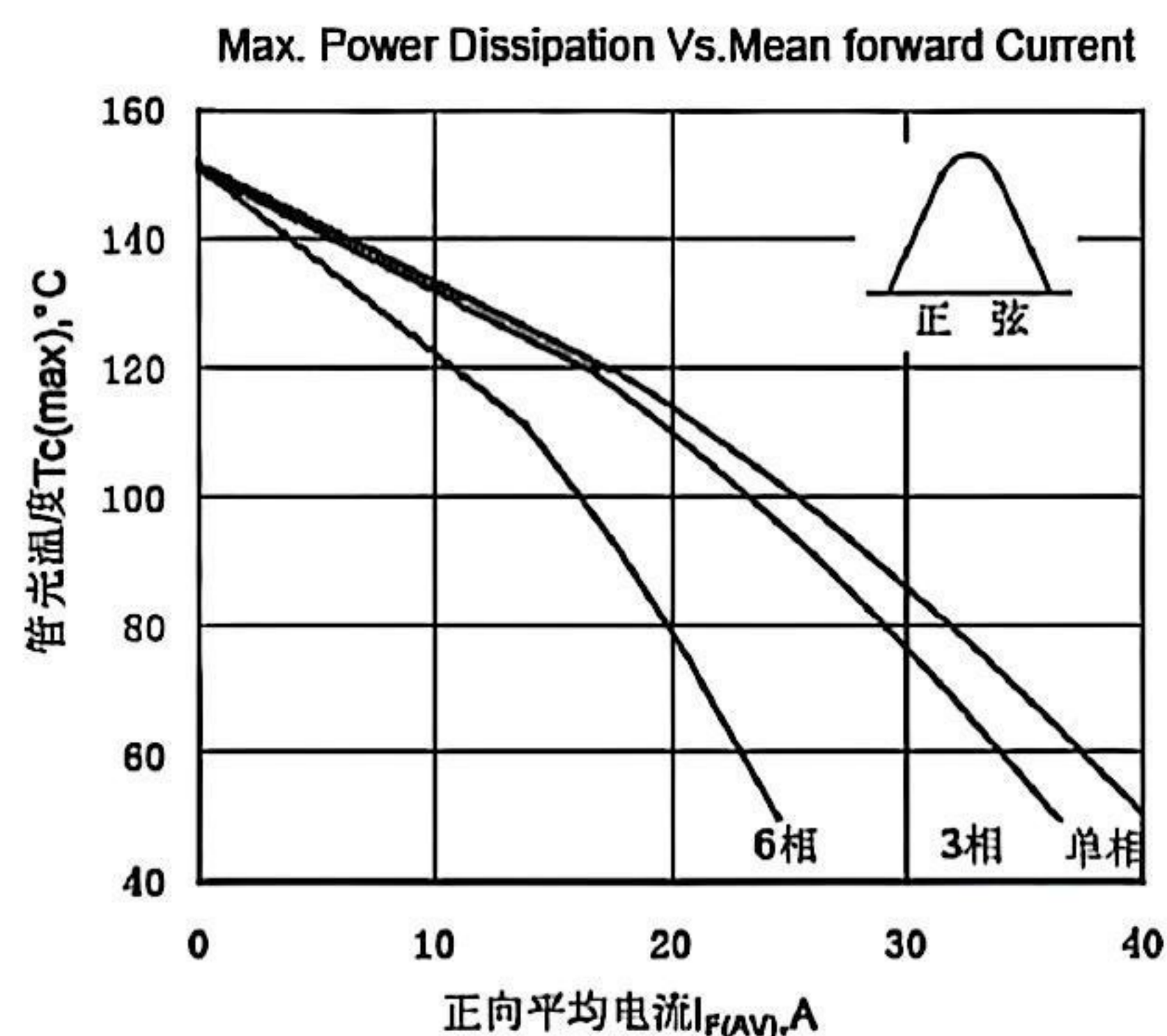
Fig.4 管壳温度与正向平均电流关系曲线
