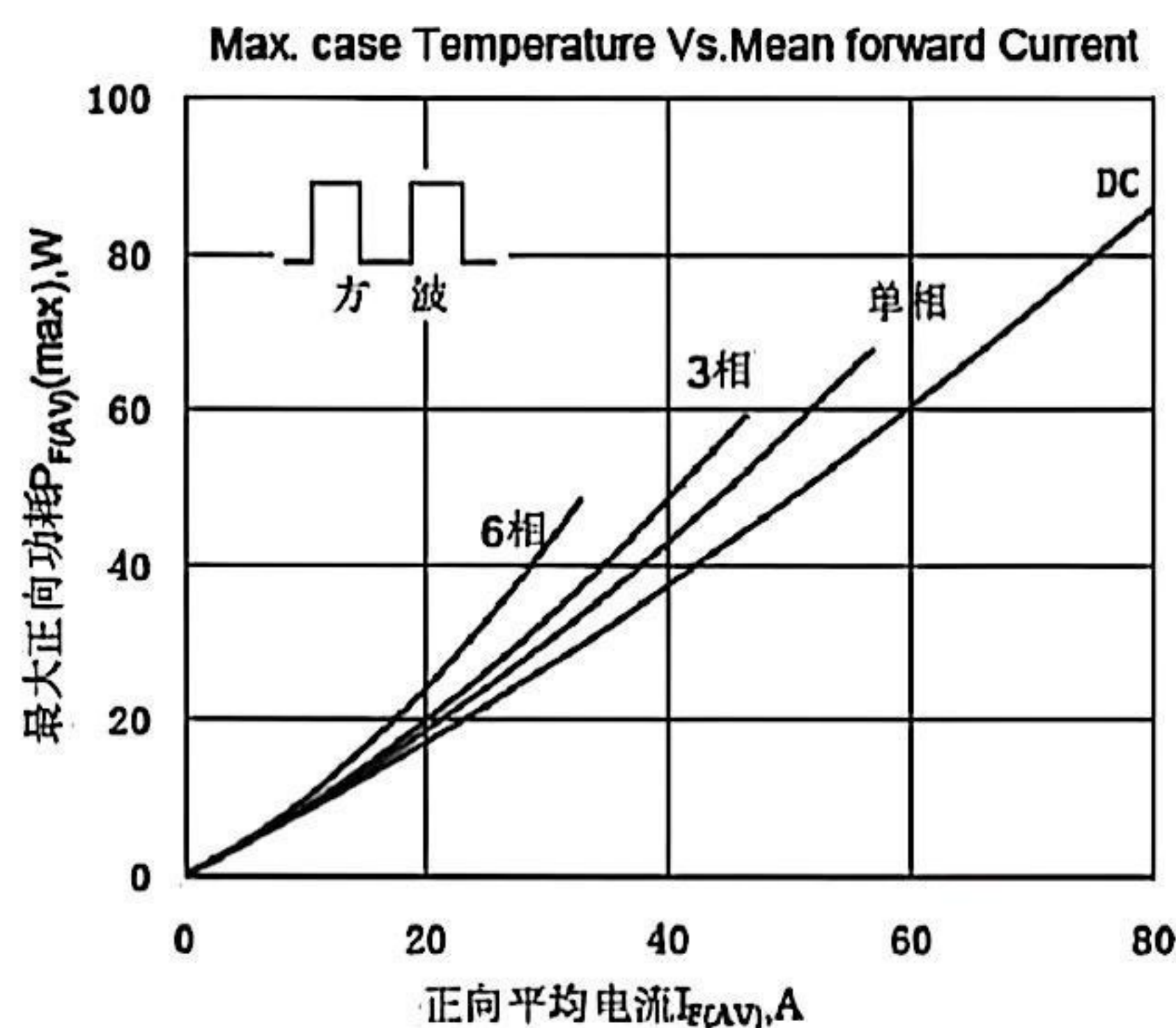
Fig.5 最大正向功耗与平均电流关系曲线
