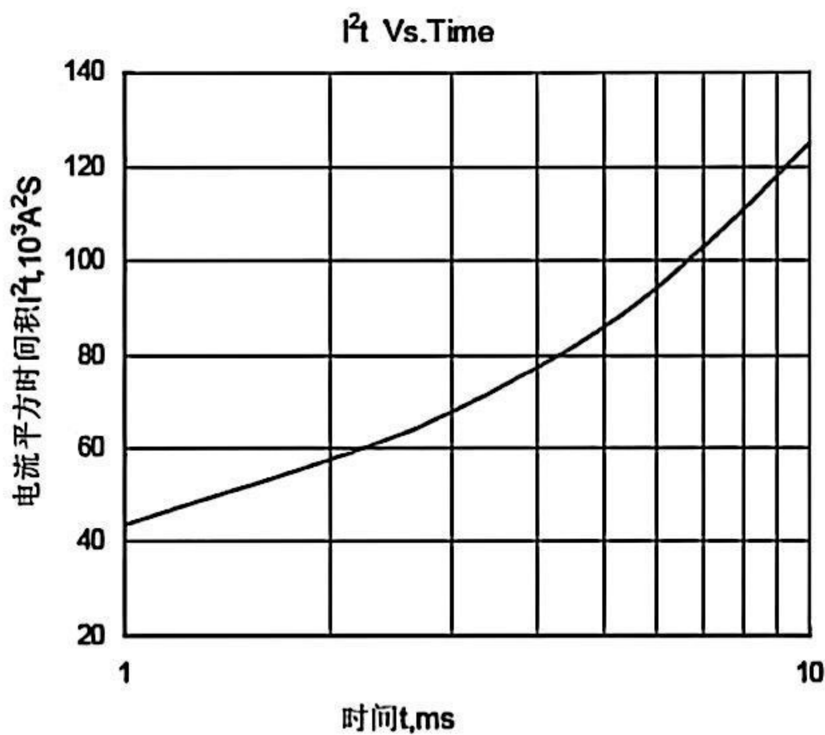
Fig.8 I^2t 特性曲线
