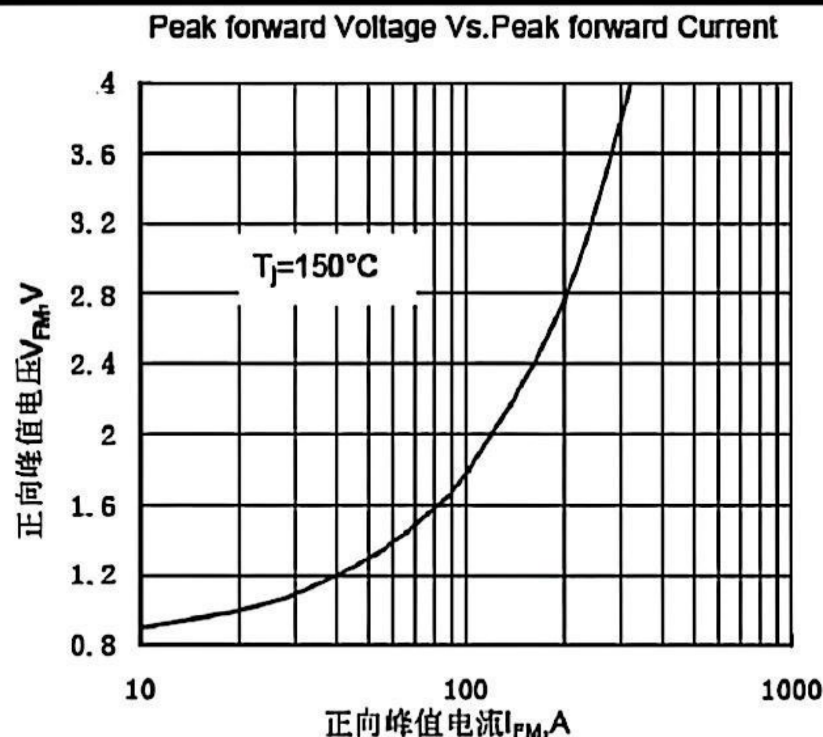
Fig.1 正向伏安特性曲线
