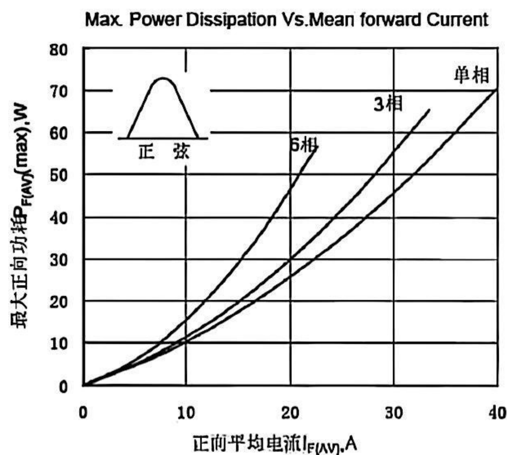
Fig.3 最大正向功耗与平均电流关系曲线
